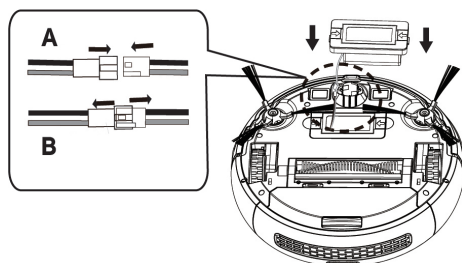
A - Połączenie terminalowe B - Odłączenie terminala ■ Czarny ■ Czerwony
