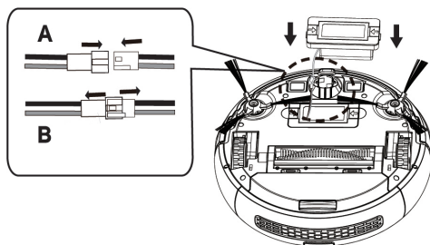
A - Conexão terminal B - Desconectando o terminal ■ Preto ■ Vermelho
