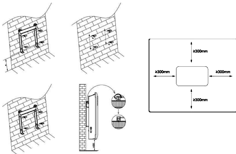
Fig.1 Instalación
